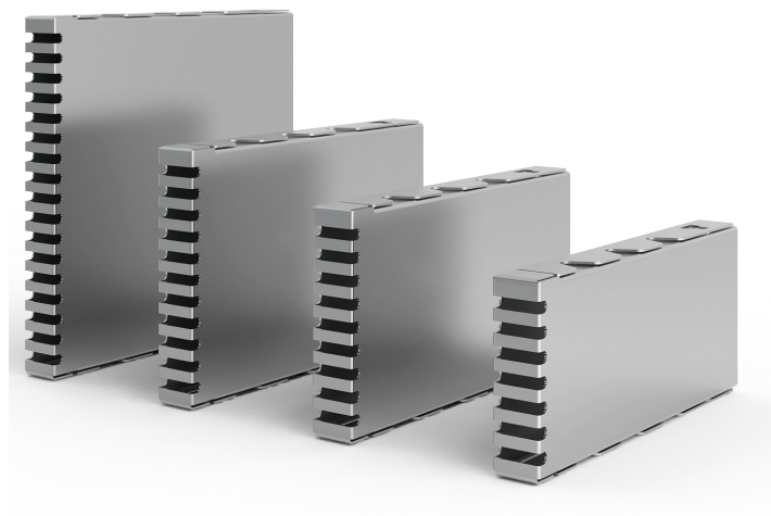
T140 voegrooster RVS standaard in vier hoogtematen; 4, 5, 6 en 9 cm
